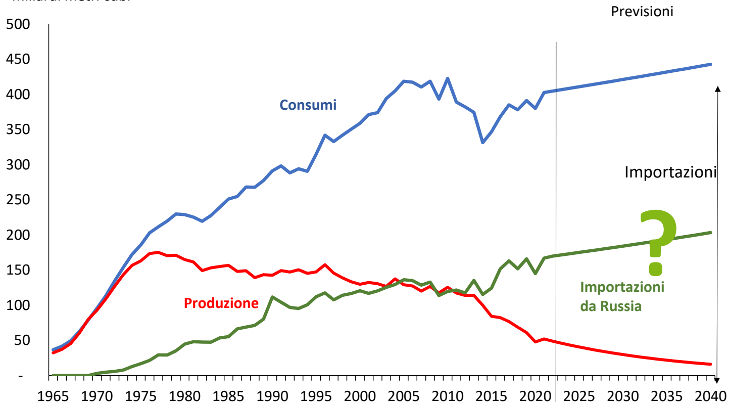
UE: importazione di gas e produzione di gas
