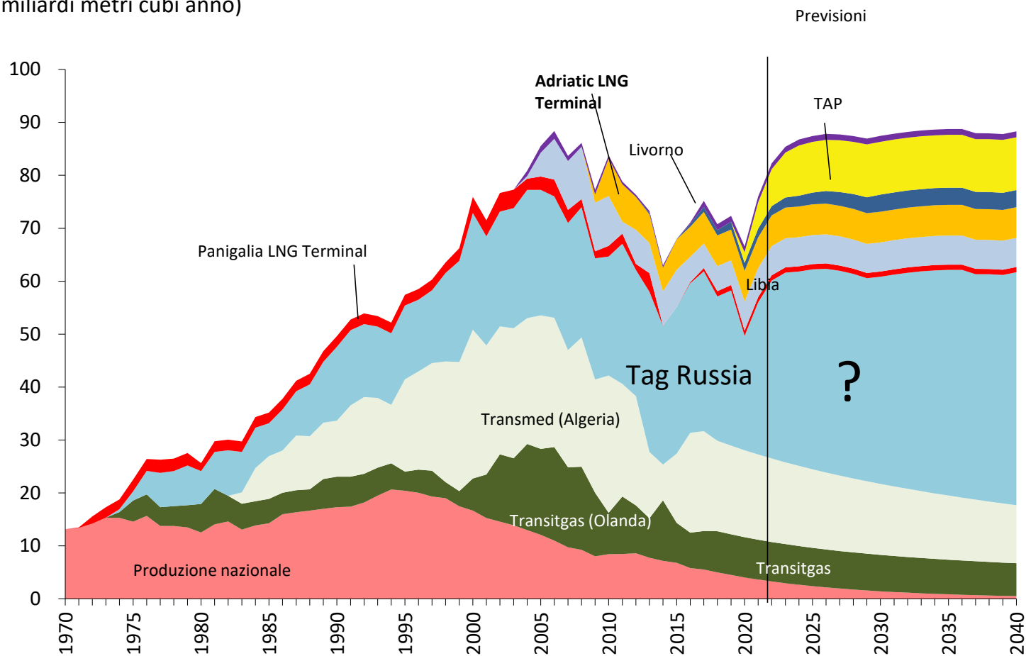
Copertura della domanda in Italia di gas (miliardi metri cubi anno)
