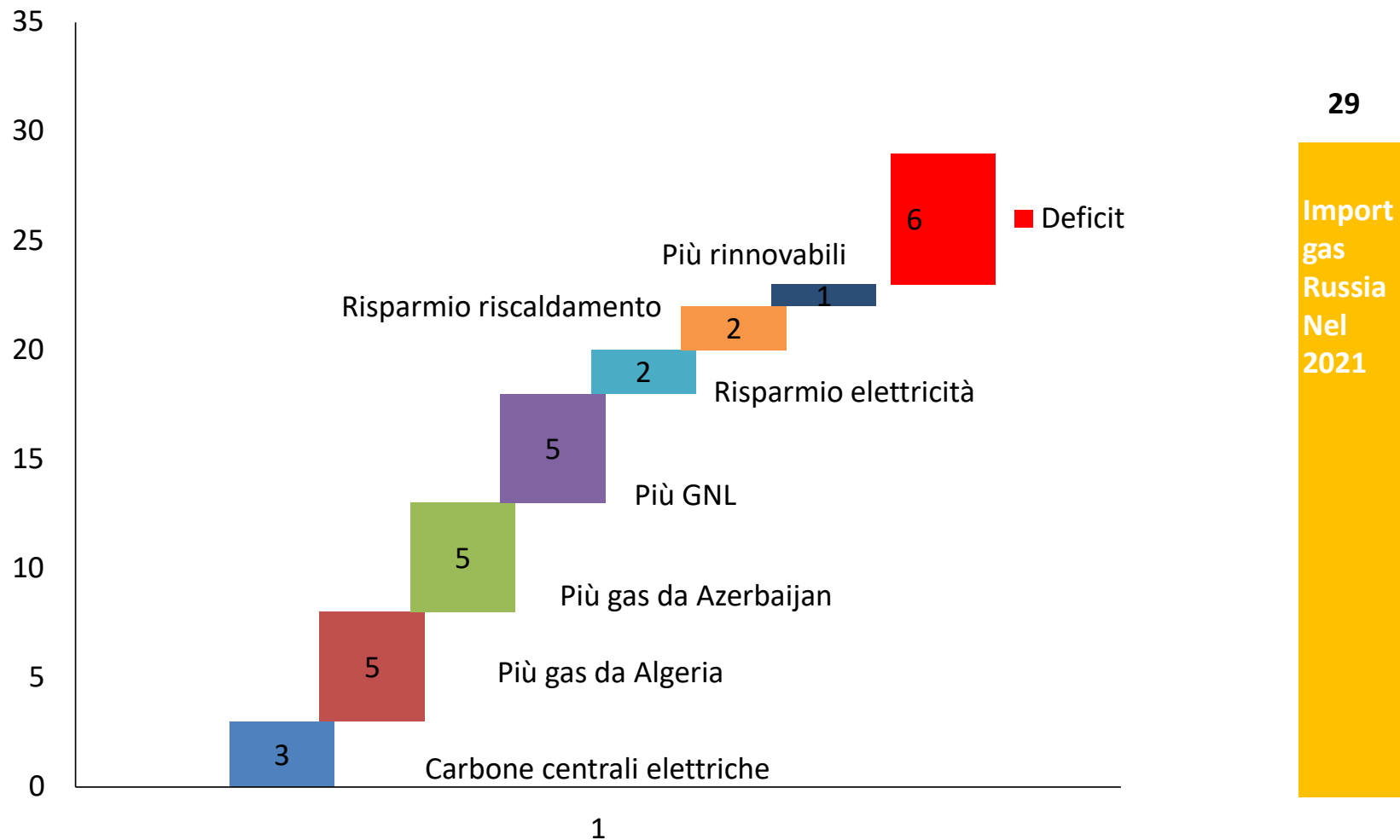
Copertura delle forniture della Russia (miliardi metri cubi)
